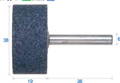
MA-861 A 36 P 回転数 24,000
